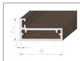
Name : Bottom beam
