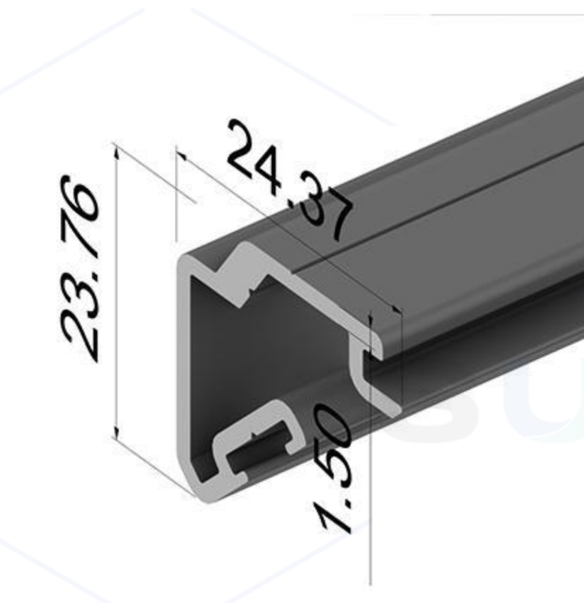
Hook
